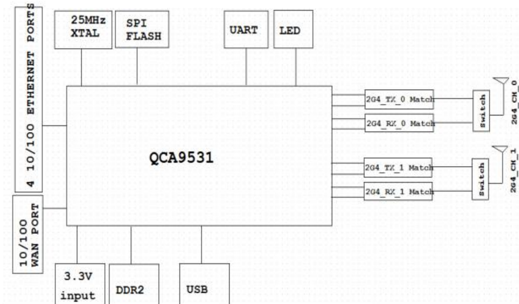
硬件框图设计
